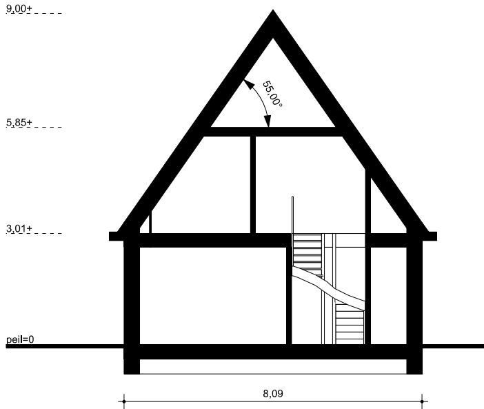
doorsnede
