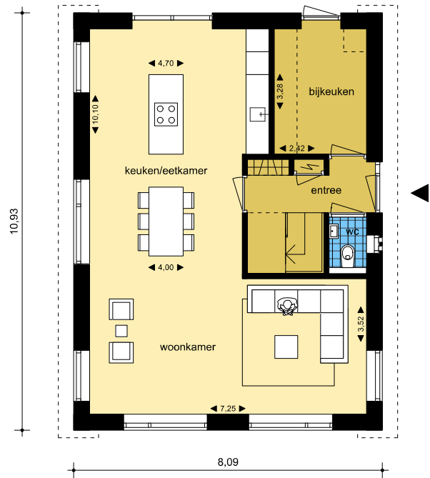
begane grond
